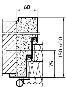
Obložková zárubeň 00/30/90 45 dB
