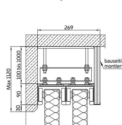
Montáž na strop zavěšená
