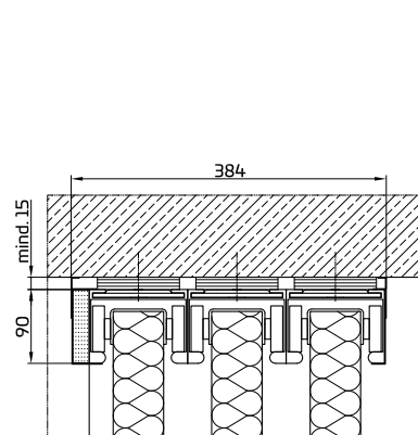
Přímá montáž na strop
