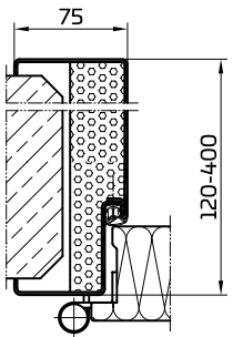
Dvoudílná obložková zárubeň 00/30 S_a/S_{200}
