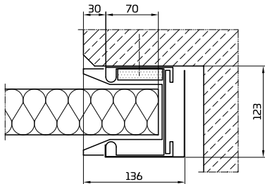
Běžné vedení Betonová stěna
