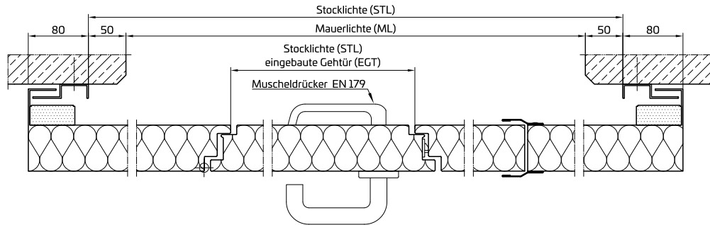
Automatická vrata dvoukřídlá s vestavěnými průchozími dveřmi, betonová stěna
