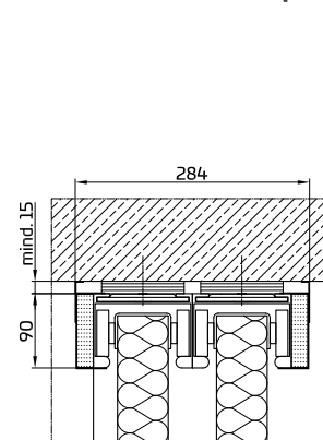
Přímá montáž na strop
