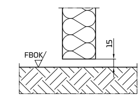
Ukončení podlahy Mezera mezi podlahou a vraty 15 mm
