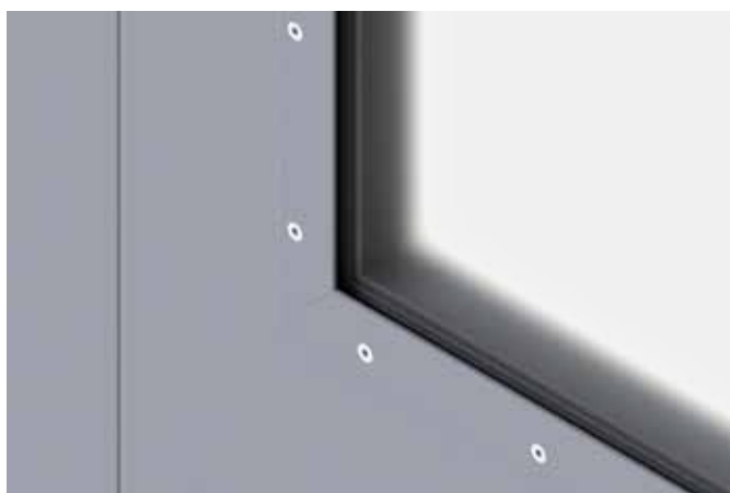
Přišroubovaná zasklívací lišta, ušlechtilá ocel, nebo prášková barva RAL dle volby
