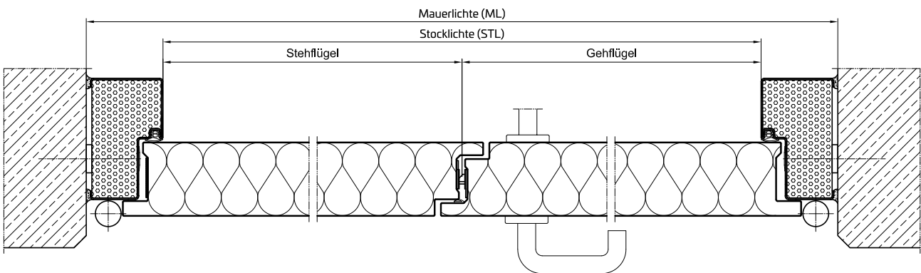
Otočné dveře dvoukřídlé s blokovou zárubní
