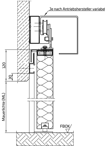
Montáž základny pohonu Rozměry se liší podle výrobce pohonu
